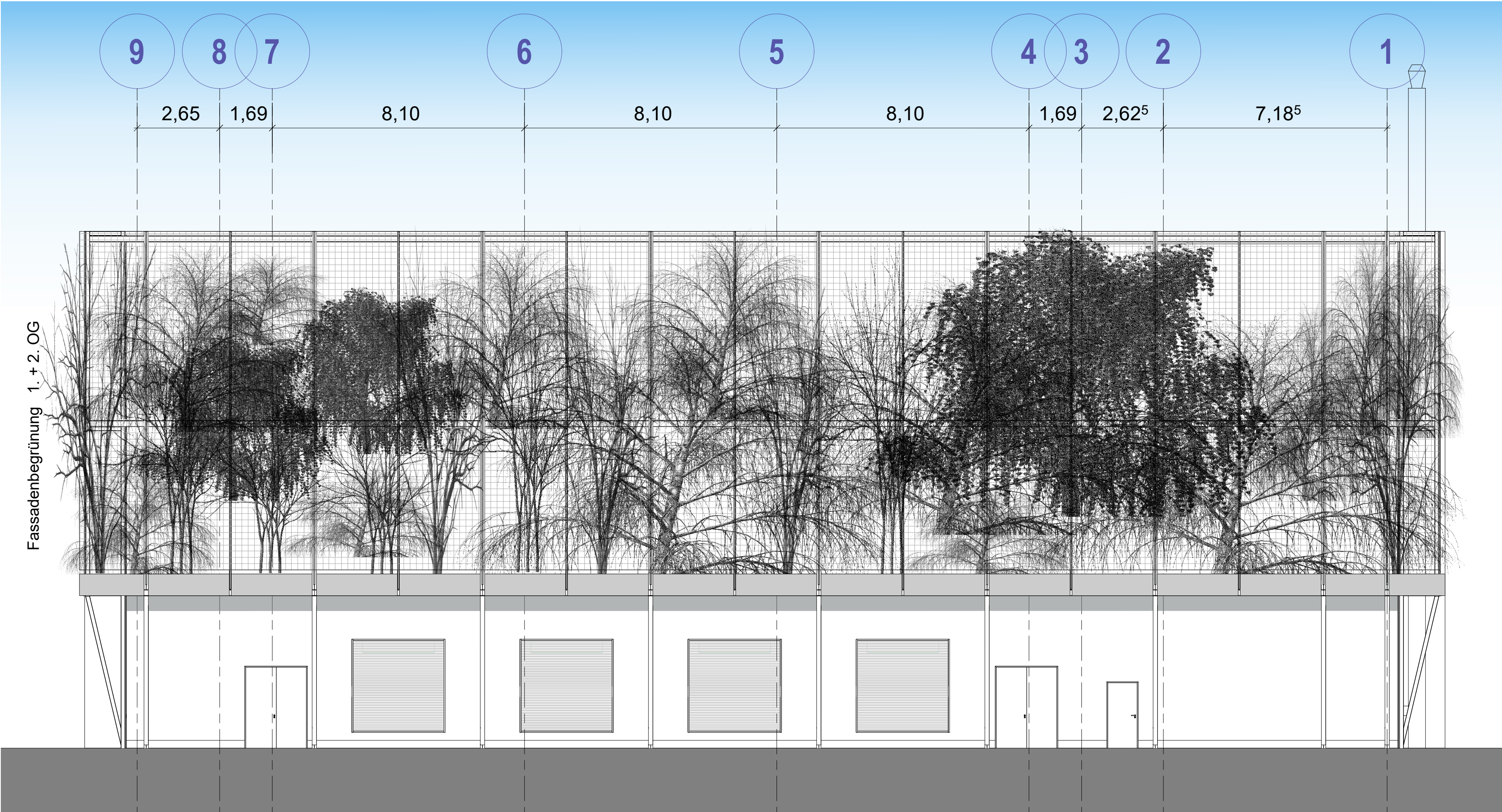
Ansicht Süd M 1:100
